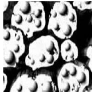
添加Outlast材料之纖維斷面圖
