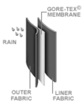
Goretex防水透濕防風示意圖
